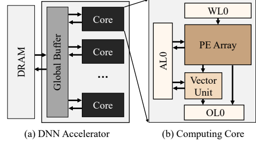
Fig. 1. DNN Accelerator Template
